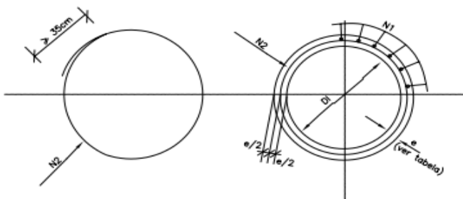
SEÇÃO TRANSVERSAL
